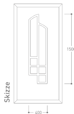
Detail Favorit 10 mit Sandstrahlglas Y 866 Float
