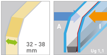
[Paneel ohne Glas bei 32 mm ca. Up 0,85, bei 34 mm ca. Up 0,79, bei 36 mm ca. Up 0,74, bei 38 mm ca. 0,70]
