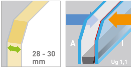
[Paneel ohne Glas bei 28 mm ca. Up 1,0, bei 30 mm ca. Up 0,9]
