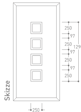
Detail Garant 13 Rahmen in Edelstahloptik
