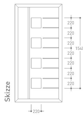
Detail Highlight 7, bündig eingelegte Edelstahlapplikationen
