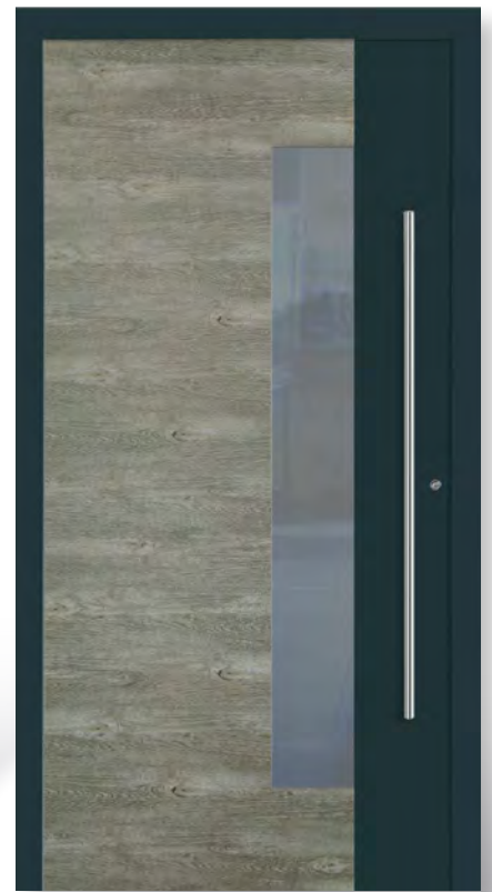
M-564 Ansicht A / DIN rechts Aufsatzfüllung inkl. Designdekor BRETT HOLZ EICHE GRAU und Applikation ähnl. RAL2 (Abb. 7016)
